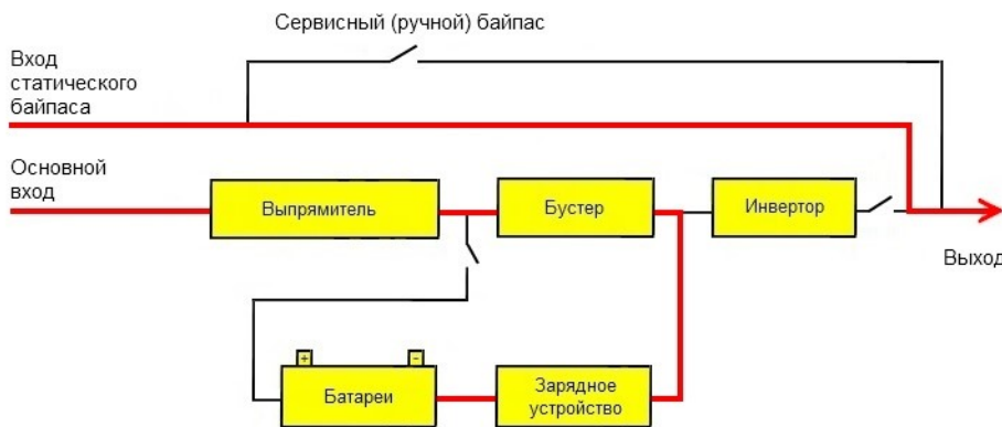
Схема работы в ЭКО режиме.
