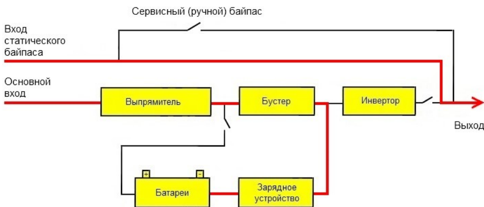
Схема работы в режиме статического байпаса
